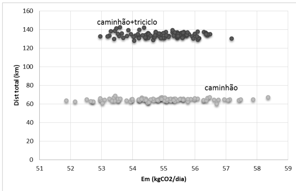
Figura 22 – Distância total versus Emissão de CO 2 .
