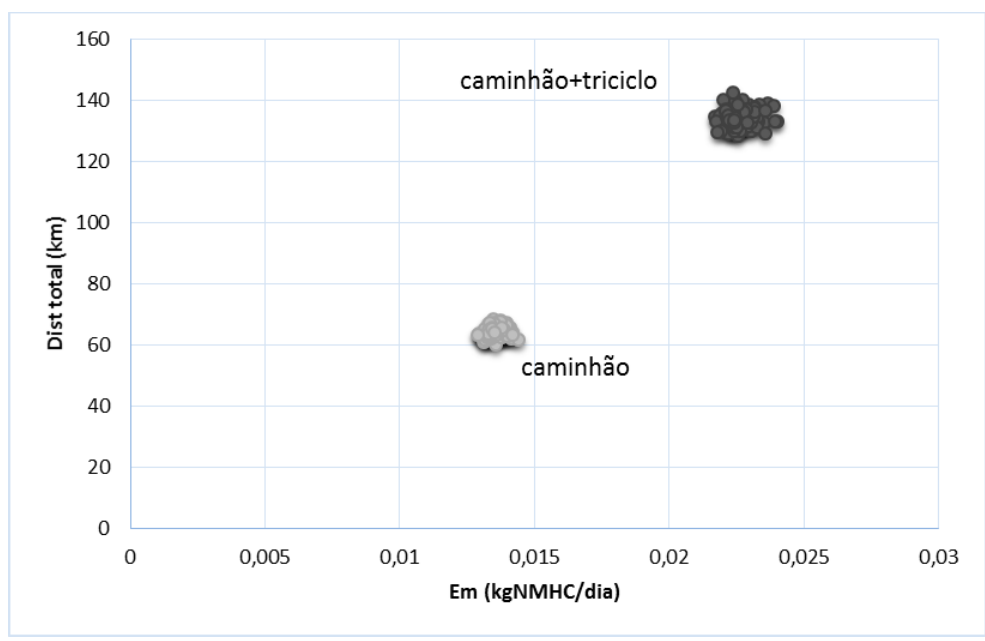
Figura 37 – Distância total versus Emissão de NMHC.
