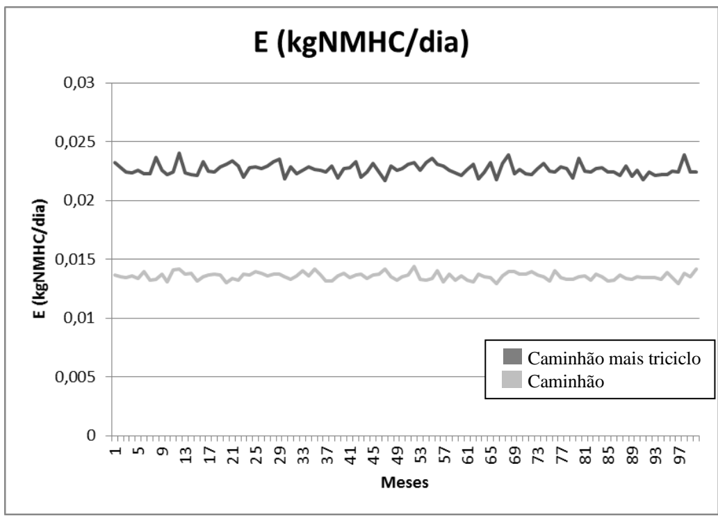
Figura 36 - Distribuição de frequência de emissão de NMHC.
