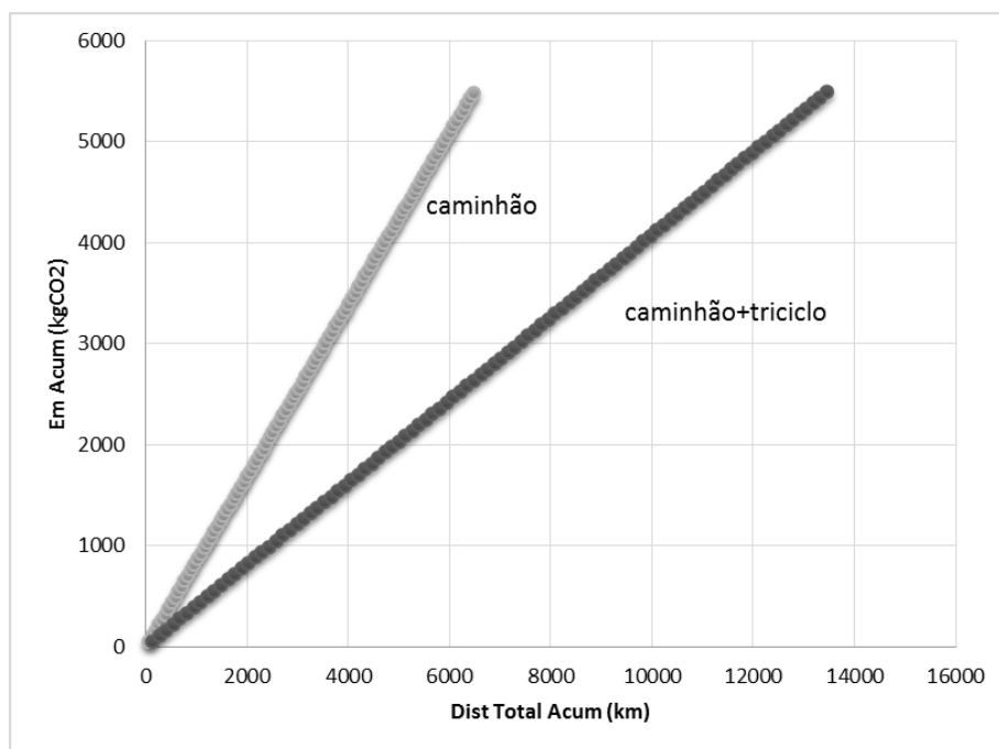
Figura 23 - Emissão de CO 2 acumulada [kg] versus Distância total acumulada [km].
