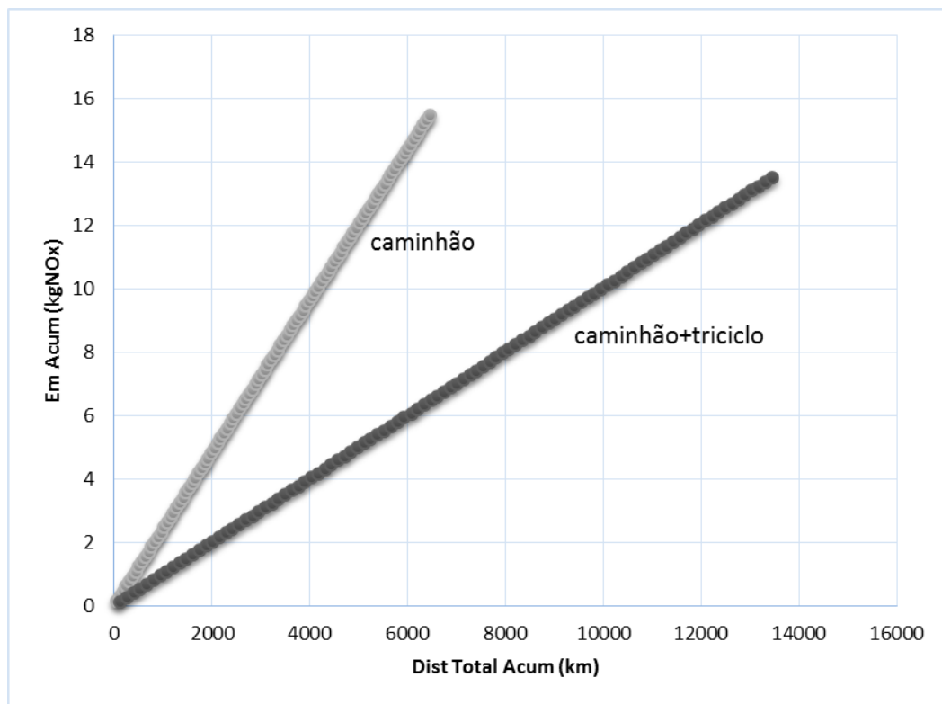
Figura 33 - Emissão de \text{NO}_x acumulada [kg] versus distância total acumulada [km].
