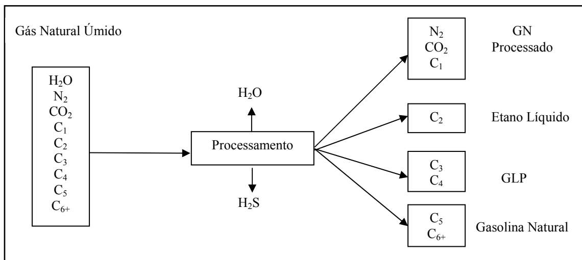
Figura 9. Resultado do processamento do gás natural na UPGN
