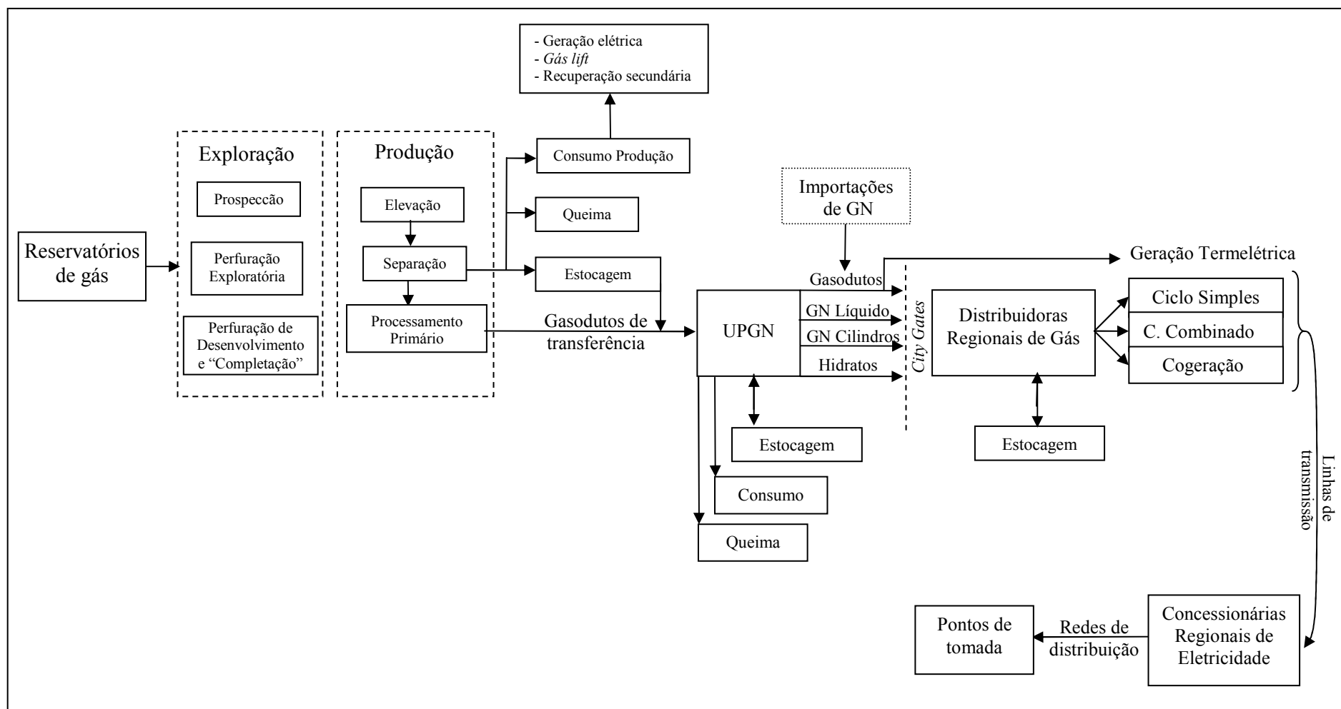
Figura 17. Fuxograma da cadeia de suprimento da energia termelétrica a gás
