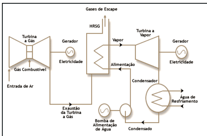
Figura 16. Fluxograma de uma termelétrica a ciclo combinado (ou fechado)
