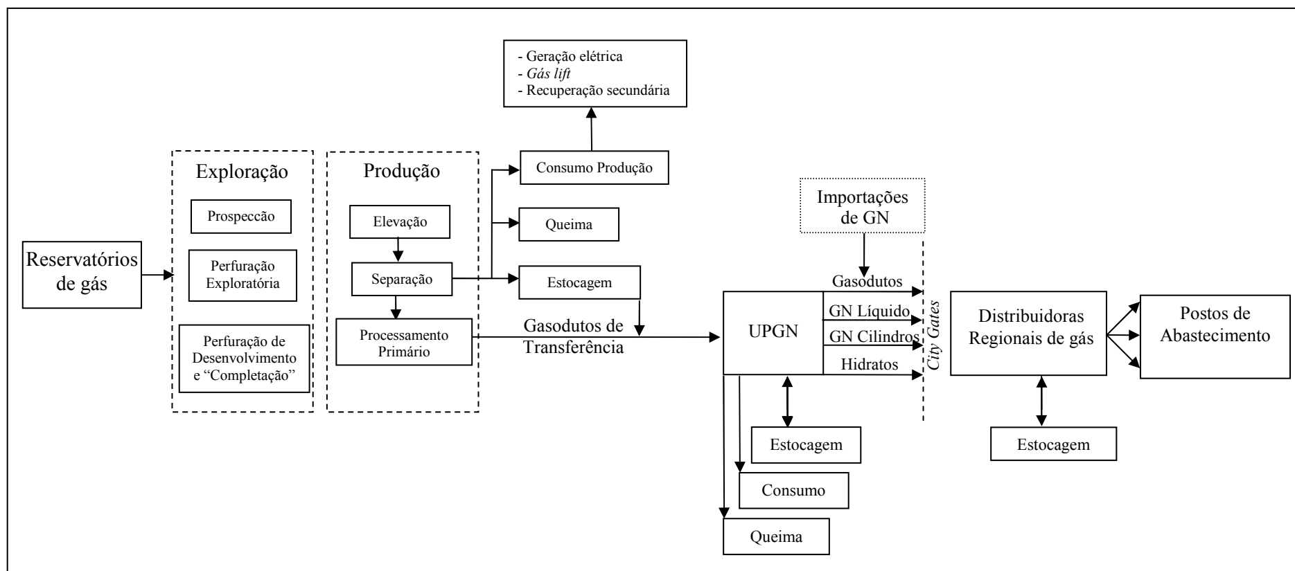
Figura 11. Fluxograma da cadeia de suprimento do gás natural comprimido
