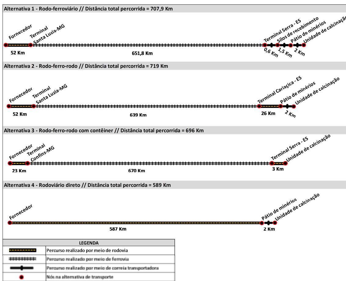
Figura 4.5 – Alternativas de transporte do calcário para abastecimento à AMT
