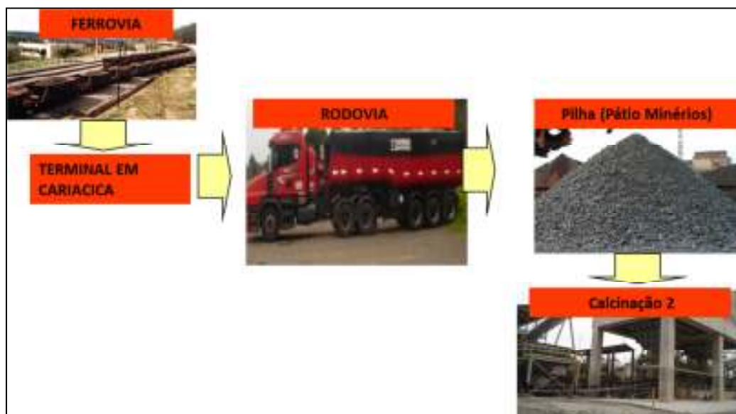
Figura 4.7 – Operação de recebimento de vagões gôndola no Terminal em Cariacica e destinação do calcário
