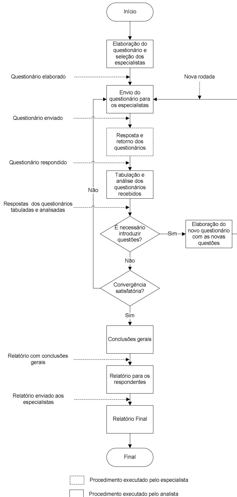
Figura 4.2 - Sequência de execução de uma pesquisa Delphi
